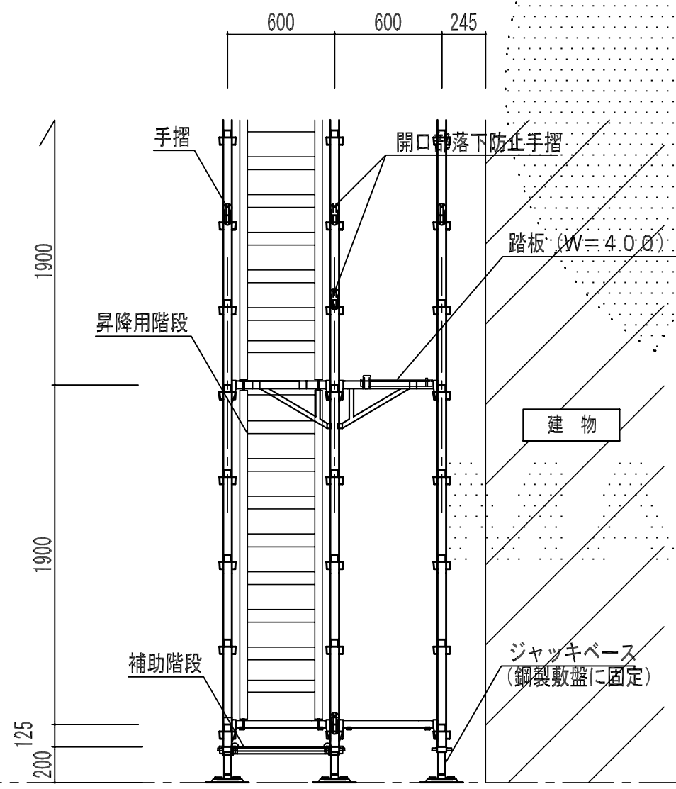
断面図 S=1/30
