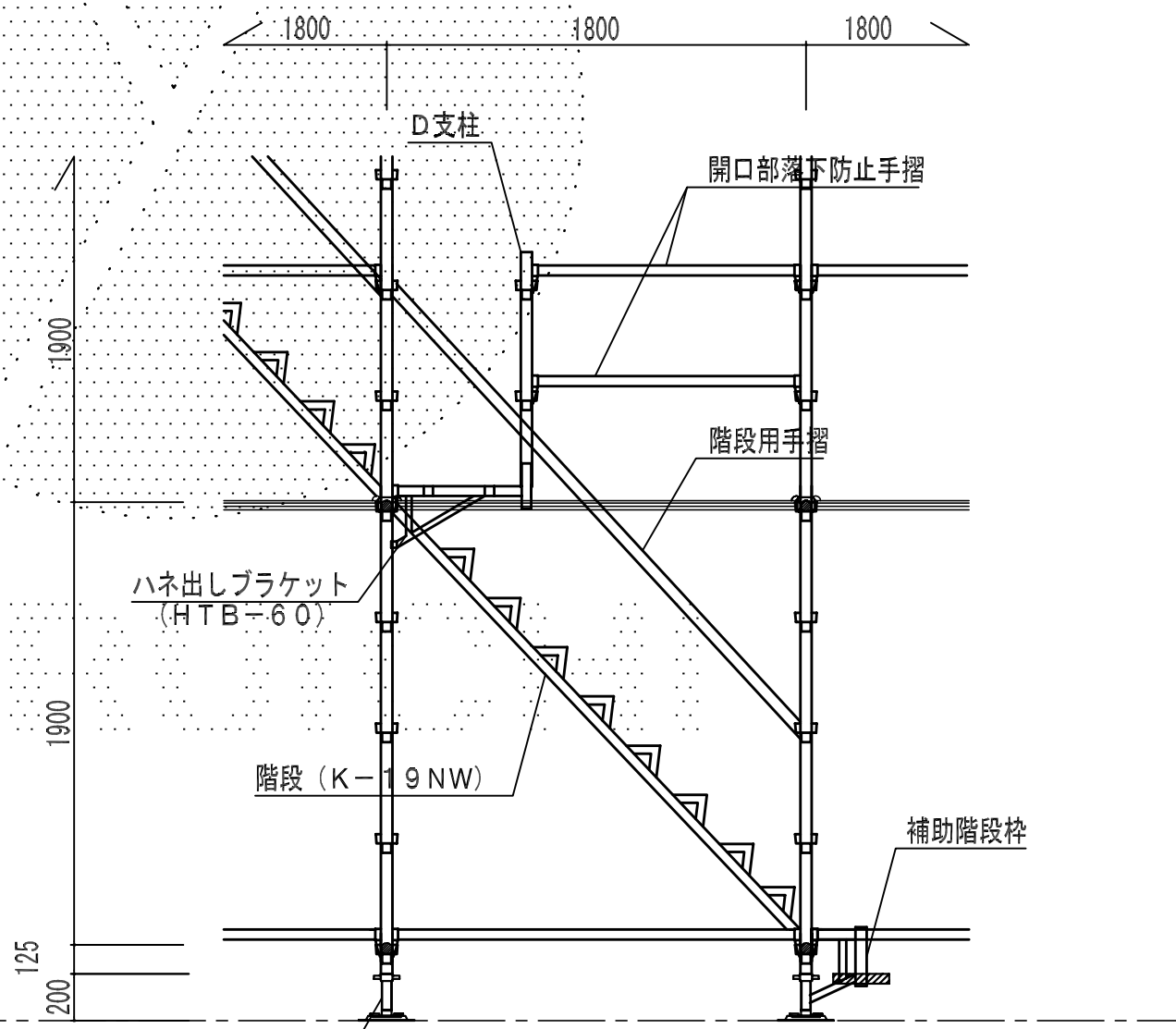
立面図 S=1/30
