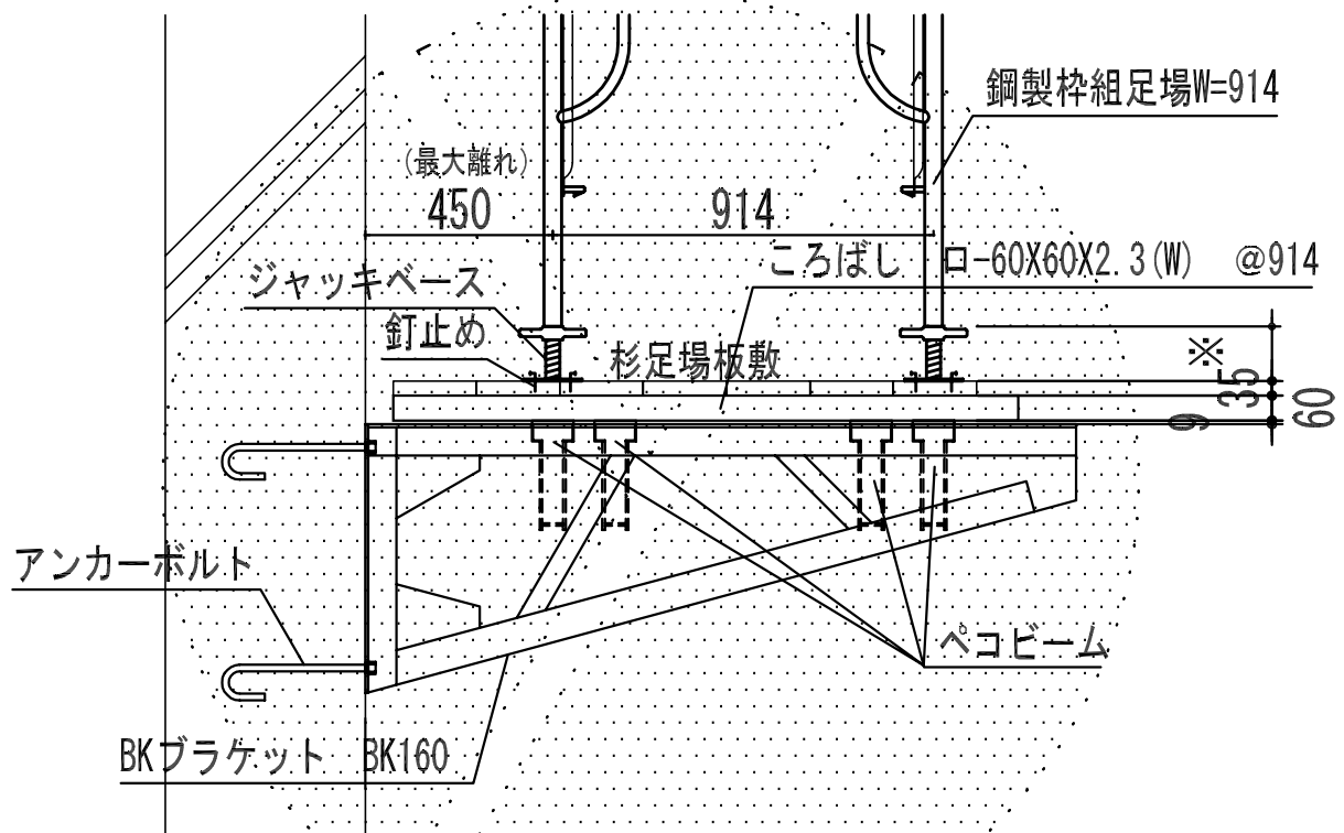
、BKブラケット使用例
