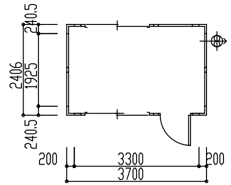
CT-37型ドア
